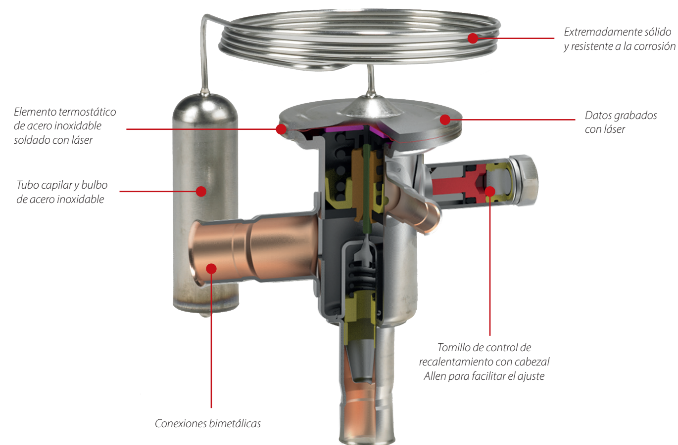
Válvula de expansión termostática TUBE
